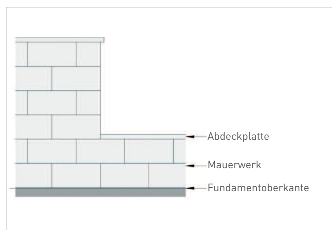
Abbildung 2: Mauerwerk
