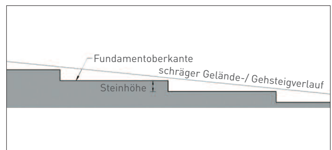
Abbildung 4: Abstufung des Fundaments gemäß Gelände-/ Gehsteigverlauf
