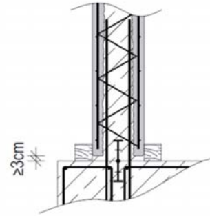
Bild 2 – Anschluss Bodenplatte/Wand
