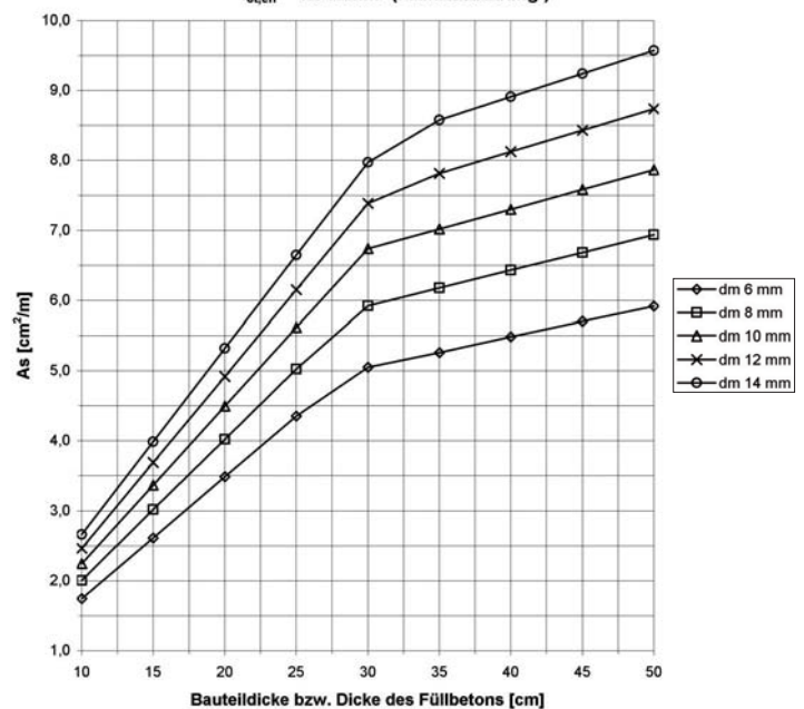
Rissebeschränkende Mindestbewehrung für zentrischen Zwang C 25/30; w_k = 0.25 mm; Betondeckung 4.0 cm; f_{ct,eff} = 1.3 N/mm 2 (Frührissbildung)
